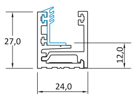
Съставен алуминиев профил
